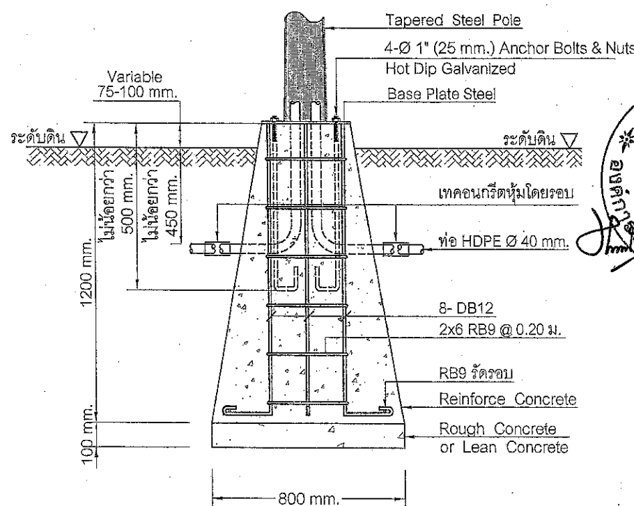
รูปตัด ①
