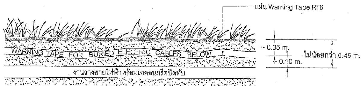
งานวางสายไฟฟ้าพร้อมเทคอนกรีตปิดทับ และ Under Ground Warning Tape
